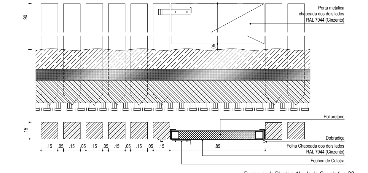
Pormenor da Planta e Alçado da Guarda tipo G2 ESC. 1:20
