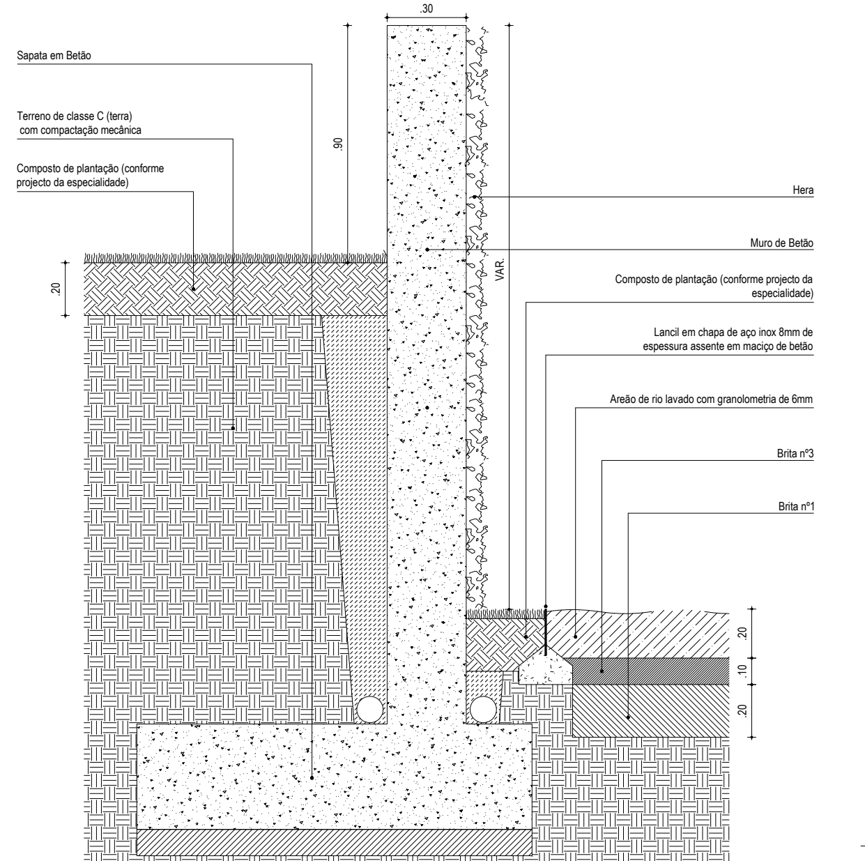
P2 Remate entre zona verde, muro de betão e zona verde ESC. 1:20
