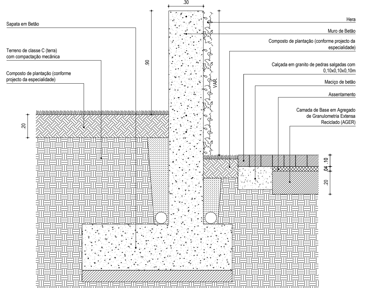
P1 Remate entre zona verde, muro de betão e rampas pedonais com betão contínuo ESC. 1:20
