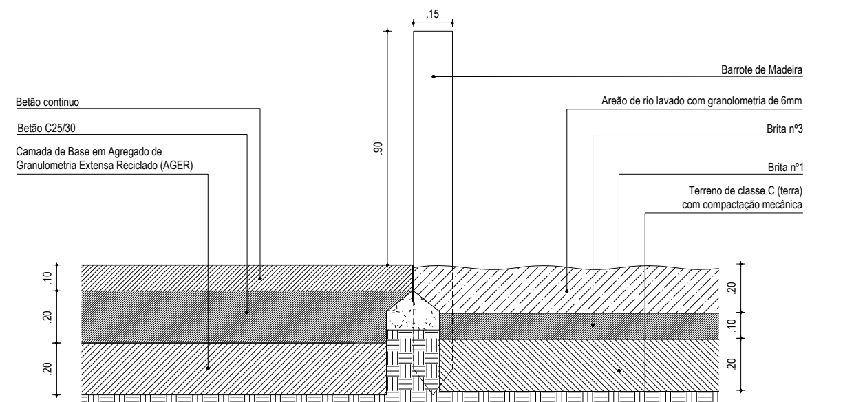
P3 Remate entre caminhos pedonais com betão contínuo, guarda em madeira G1 e zona de areão ESC. 1:20
