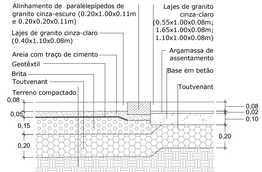
P13 - Alinhamento de paralelepípedos de granito cinza-escuro entre pavimentos automóvel ligeiro e pedonal em lajes de granito cinza-claro (0.40x1.10x0.08m e 0.55x1.00x0.08m; 1.65x1.00x0.08m; 1.10x1.00x0.08m) Corte transversal
