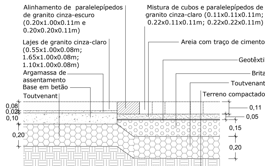
P7 - Alinhamento de paralelepípedos de granito cinza-escuro entre pavimento automóvel e pedonal composto por mistura de cubos e paralelepípedos de granito cinza-claro e pavimento automóvel ligeiro e pedonal em lajes de granito cinza-claro de grandes dimensões Corte transversal
