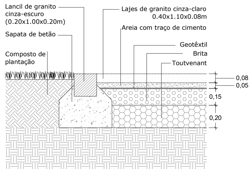
P16 - Remate entre pavimento automóvel ligeiro e pedonal em lajes de granito cinza-claro de 0.40x1.10m e zona verde Corte transversal
