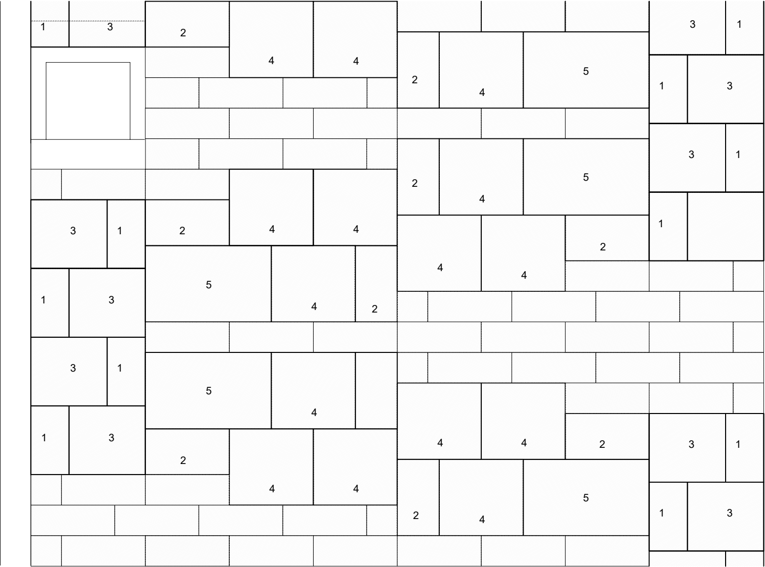
P 40 - Estereotomia dos pavimentos das rampas em lajes de granito cinza-claro (dimensões 1_0.50x0.90x0.05m; 2_0.60x1.10x0.05m; 3_1.00x0.90x0.05m; 4_1.10x1.00x0.05m; 5_1.65x1.00x0.05m) e do revestimento dos cobertores dos degraus em lajes boleadas de granito cinza-claro (0.43x1.10x0.05m) Planta 1/50
