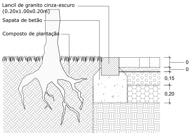
P6 - Lancil de granito cinza-escuro entre pavimento automóvel e pedonal composto por mistura de cubos e paralelepípedos de granito cinza-claro e caldeira Corte transversal
