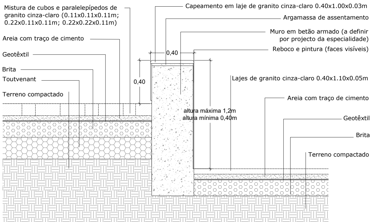
P30 - Muro de remate entre escada/rampa de acesso à Igreja e a faixa automóvel . Corte transversal
