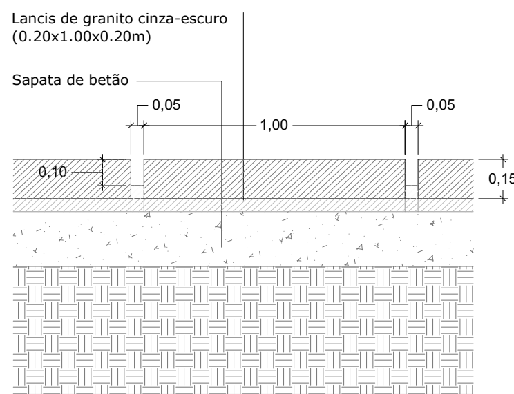
P3 - Remate descontinuo em lancis de granito cinza-escuro entre zona verde e pavimento automóvel e pedonal composto por mistura de cubos e paralelepípedos de granito cinza-claro Corte longitudinal
