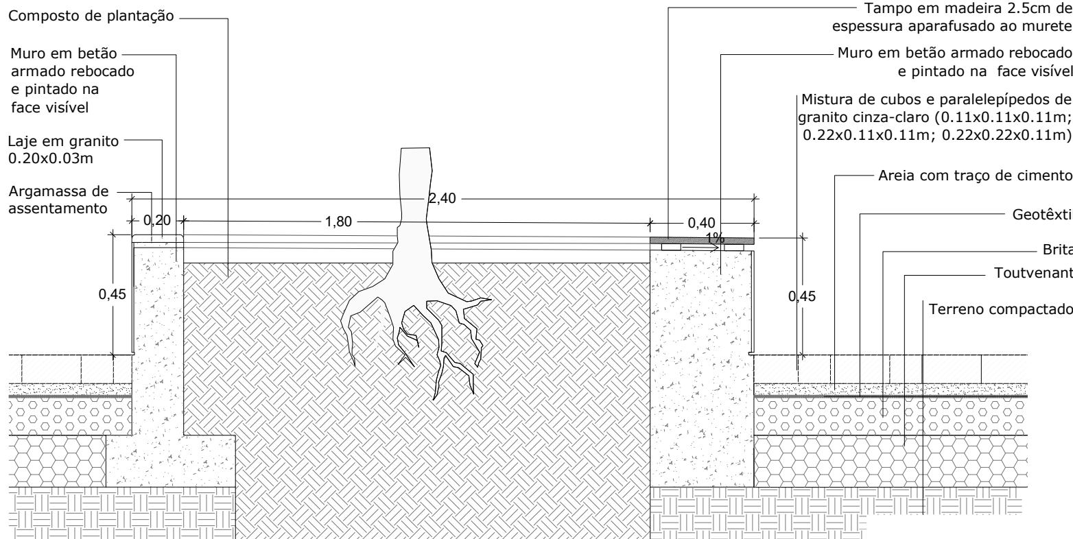
P33 - Caldeira sobreelevada para árvore, capeada a lajes de granito cinza-claro e com banco em tampo de madeira. Corte transversal
