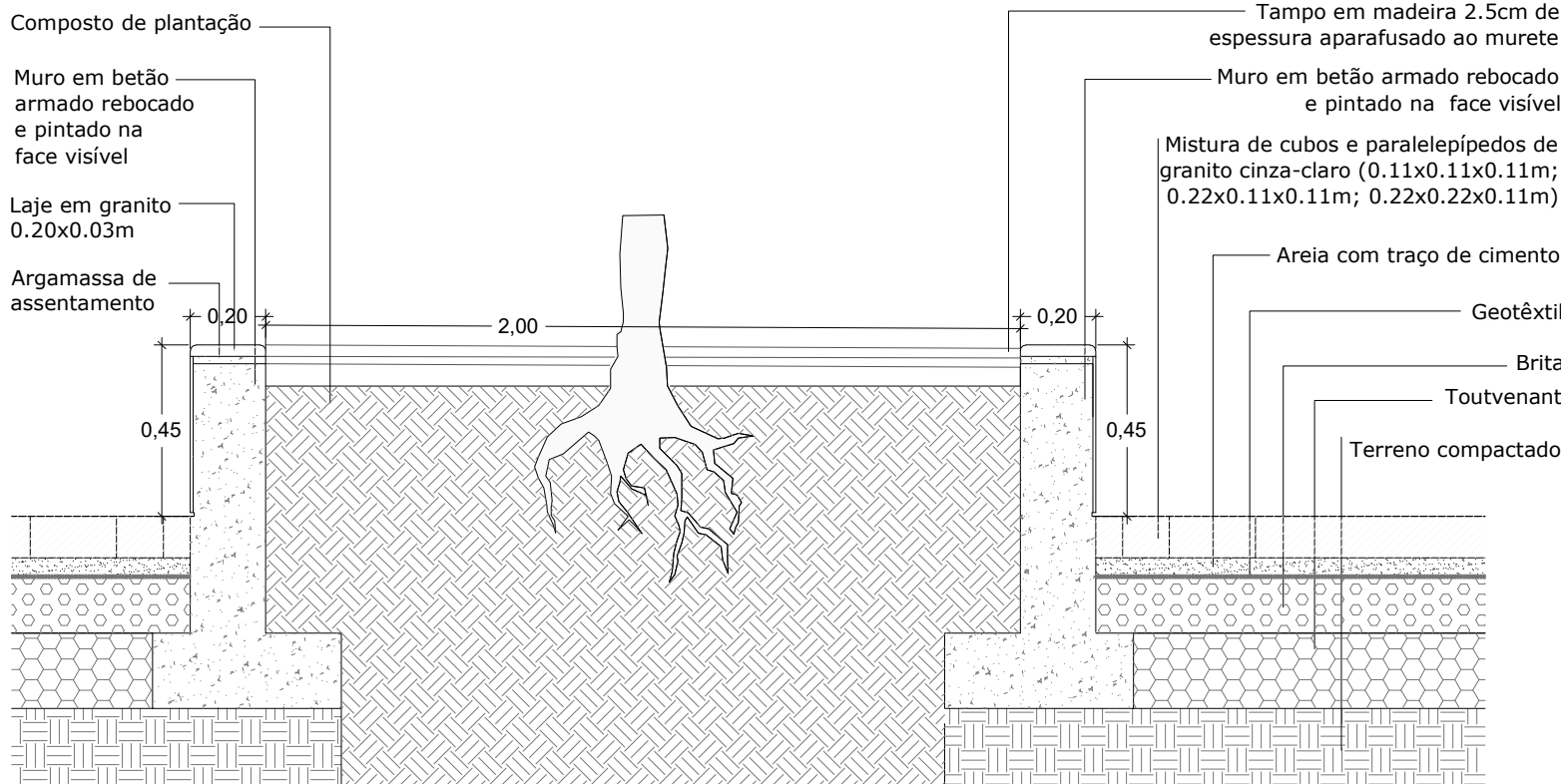
P32 - Caldeira sobreelevada para árvore, capeada a lajes de granito cinza-claro Corte transversal
