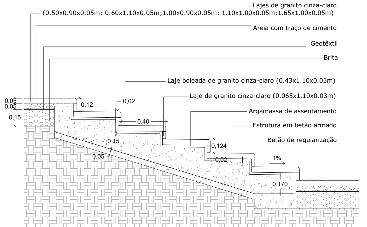
P26 - Escada em betão armado com revestimento a lajes de granito cinza-claro (dimensões 0.43x1.10x0.05m e 0.065x1.10x0.03m (espelho)) Corte transversal
