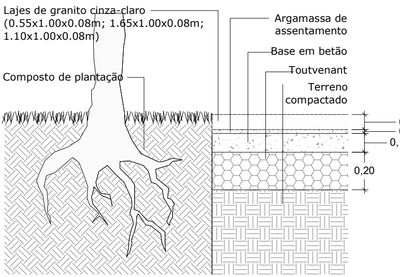
P18 - Remate entre pavimento automóvel ligeiro e pedonal em lajes de granito cinza-claro de grandes dimensões e caleira Corte transversal
