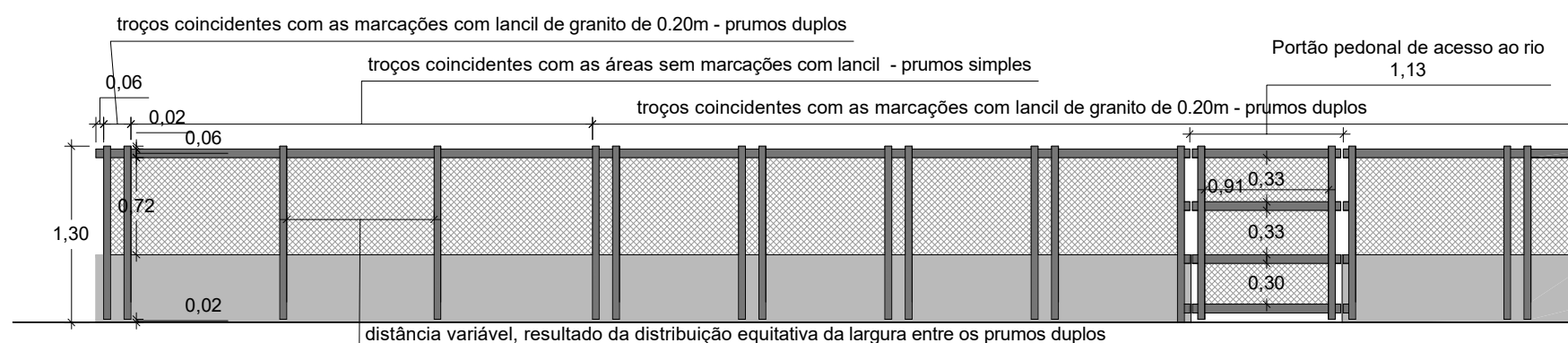
P46 - Guarda e porta de homem 4 de abrir em prumos e tubos metálicos, com revestimento em rede em aço inoxidável.
