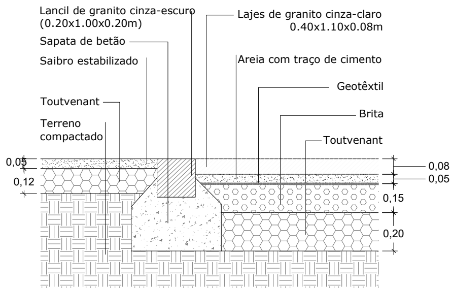
P20 - Lancil de granito cinza-escuro entre pavimento automóvel ligeiro e pedonal em lajes de granito cinza-claro de 0.40x1.10m e pavimento em saibro Corte transversal
