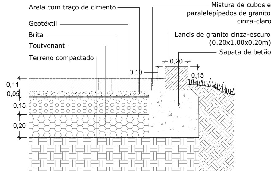
P3 - Remate descontinuo em lancis de granito cinza-escuro entre zona verde e pavimento automóvel e pedonal composto por mistura de cubos e paralelepípedos de granito cinza-claro Corte transversal
