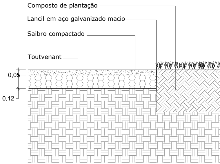
P23 - Lancil em aço entre pavimento em saibro e zona verde Corte transversal
