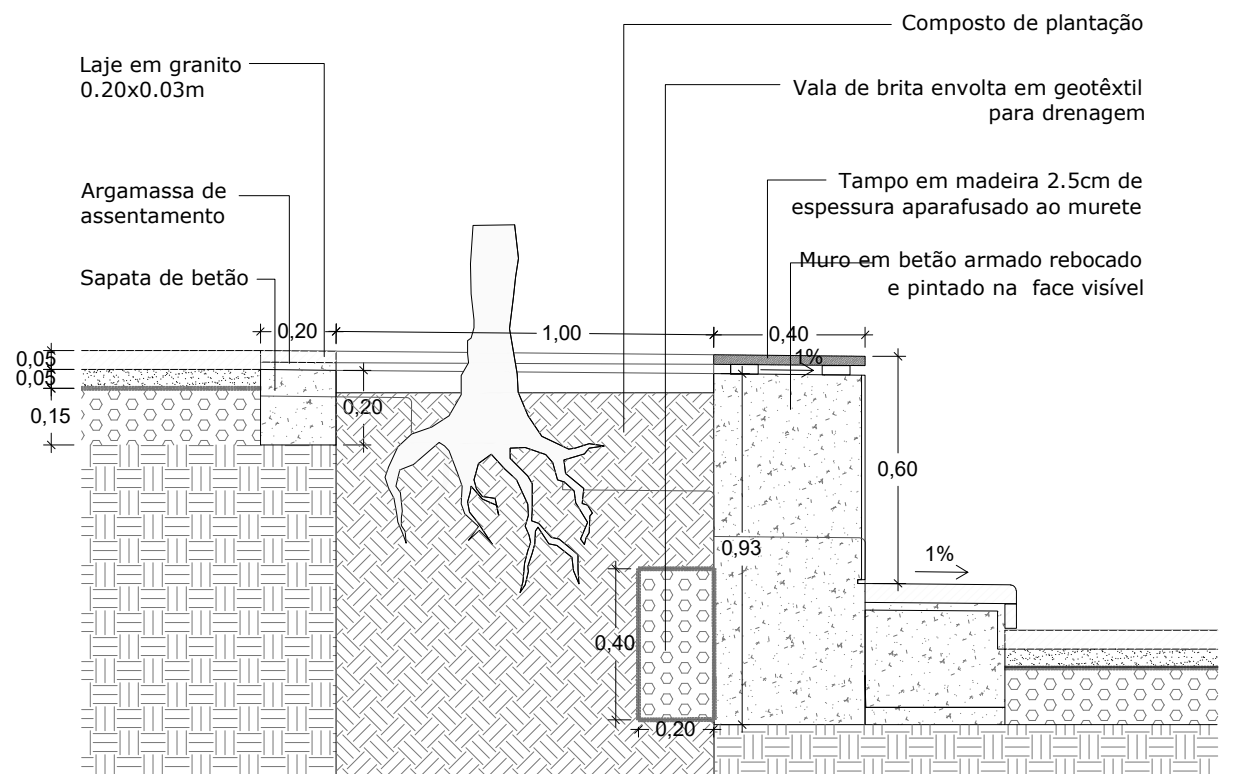
P28 - Caldeira para árvore, encaixada na escada, capeada a lajes de granito cinza-claro e banco em tampo de madeira. Corte transversal
