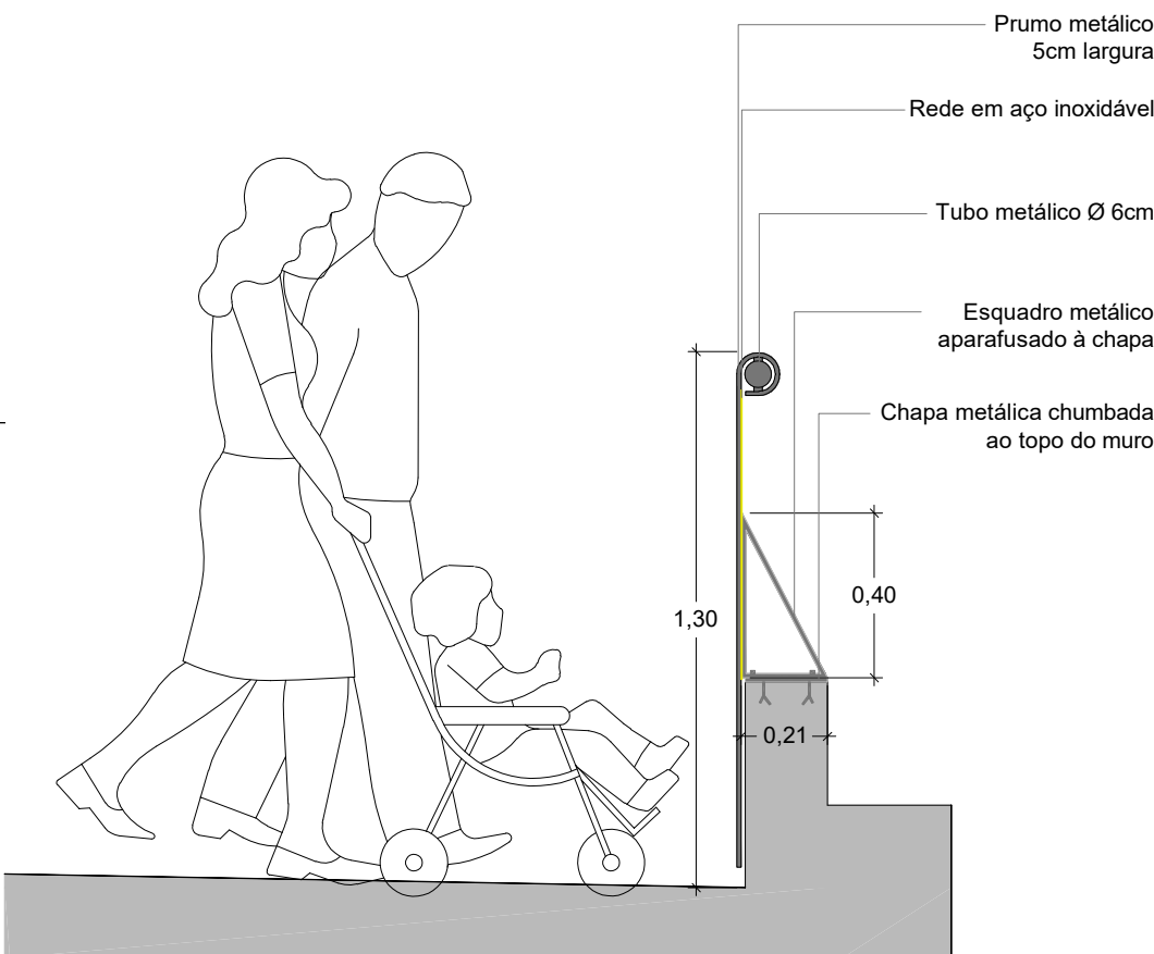
P44 - Guarda em prumos e tubos metálicos, com revestimento em rede em aço inoxidável.
