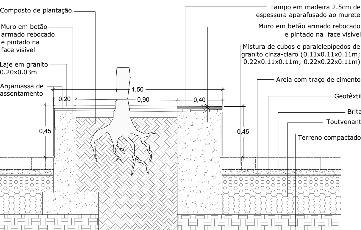
P31 - Caldeira sobreelevada para árvore, capeada a lajes de granito cinza-claro e com banco em tampo de madeira. Corte transversal
