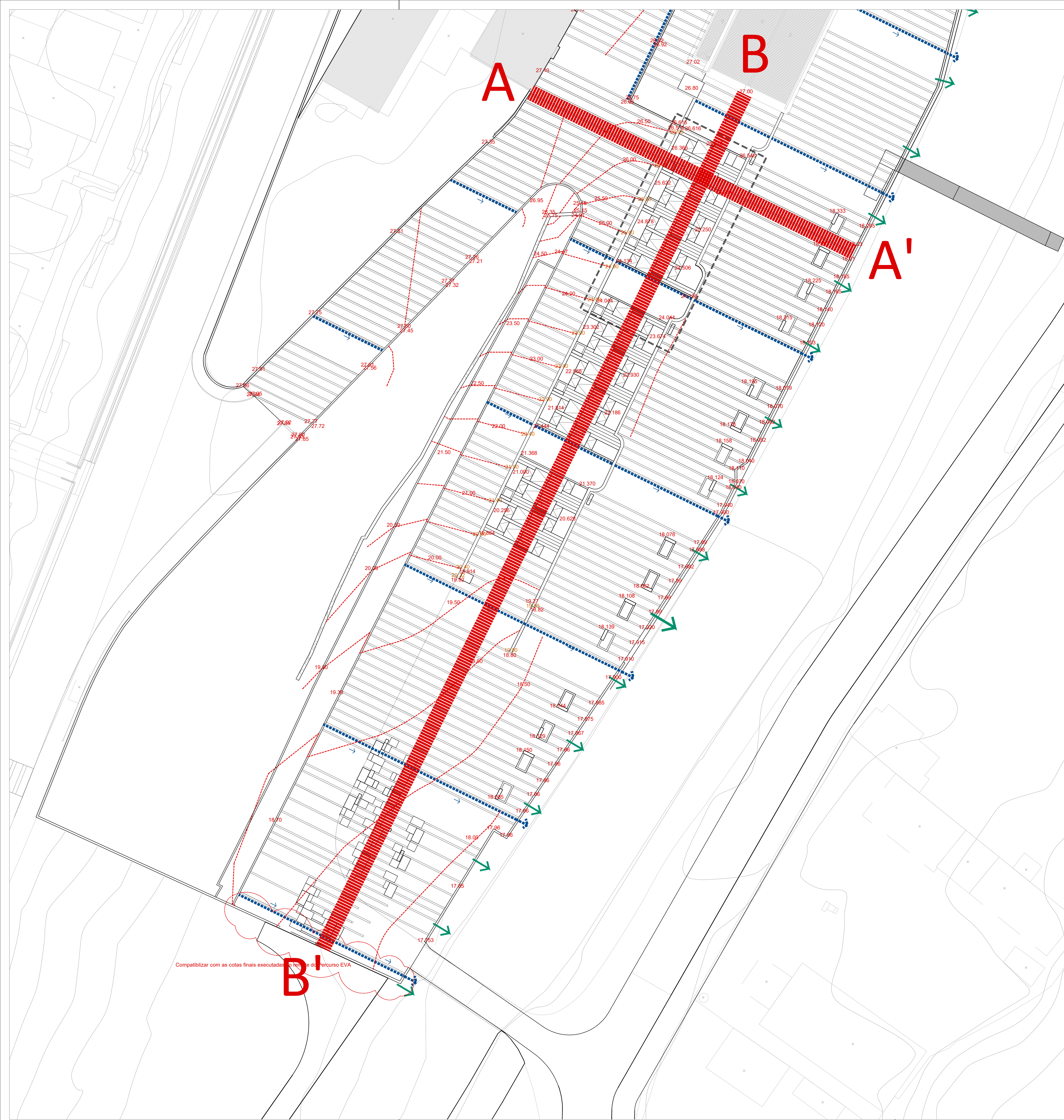
Implantação altimétrica da escada/rampa - detalhe, esc. 1/75
