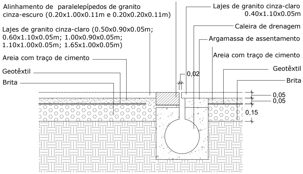
P25 - Alinhamento de paralelepípedos de granito cinza-escuro e caleira de drenagem entre rampas em lajes de granito cinza claro e patamares em lajes de granito cinza-claro de 0.40x1.10x0.05m Corte transversal
