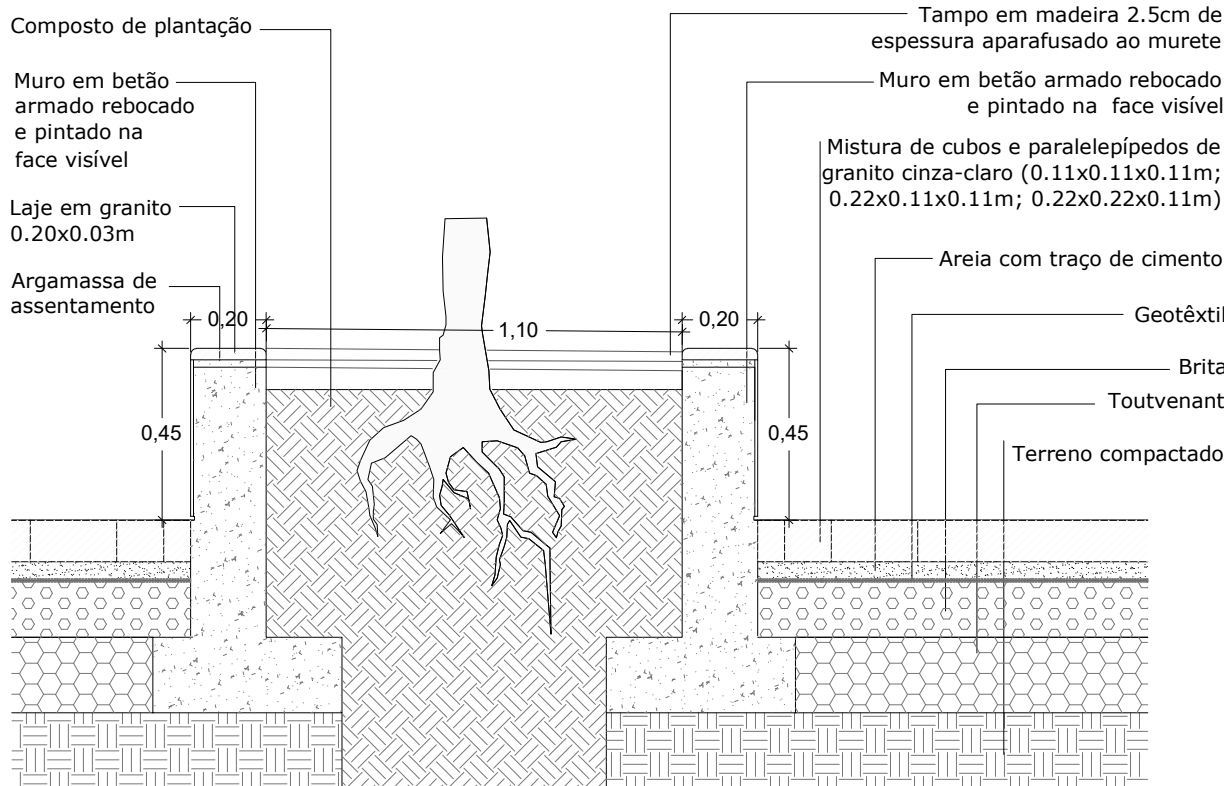
P34 - Caldeira sobreelevada para árvore, capeada a lajes de granito cinza-claro Corte transversal
