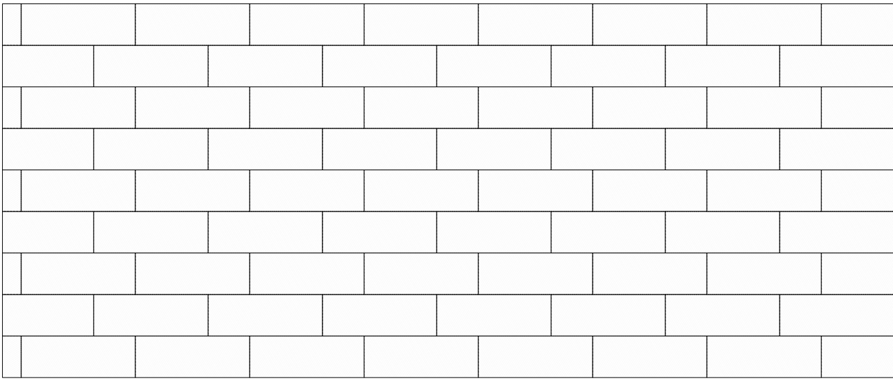
P 41 - Estereotomia dos pavimentos automóvel ligeiro e pedonal em lajes de granito cinza-claro com as dimensões 0.40x1.10x0.08/0.05m Planta 1/50
