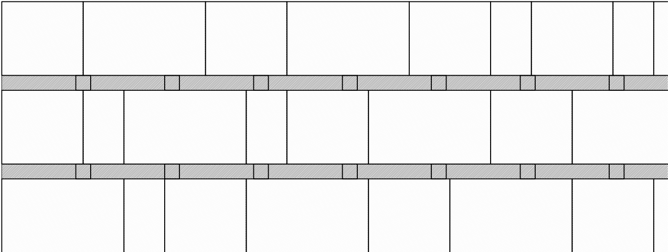
P 39 - Estereotomia dos pavimentos automóvel ligeiro e pedonal em lajes de granito cinza-claro (dimensões: 0.55x1.00x0.08/0.05m; 1.65x1.00x0.08/0.05m; 1.10x1.00x0.08/0.05m) com alinhamentos de paralelepípedos de granito cinza-escuro (0.20x1.00x0.11m e 0.20x0.20x0.11m) Planta 1/50
