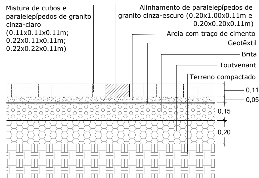
P1 - Alinhamento de paralelepípedos de granito cinza-escuro em pavimento automóvel e pedonal composto por mistura de cubos e paralelepípedos de granito cinza-claro Corte transversal
