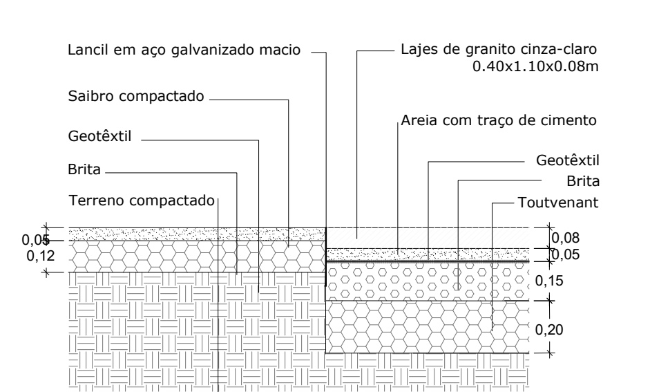
P22 - Lancil em aço entre pavimento automóvel ligeiro e pedonal em lajes de granito cinza-claro de 0.40x1.10m e pavimento em saibro Corte transversal
