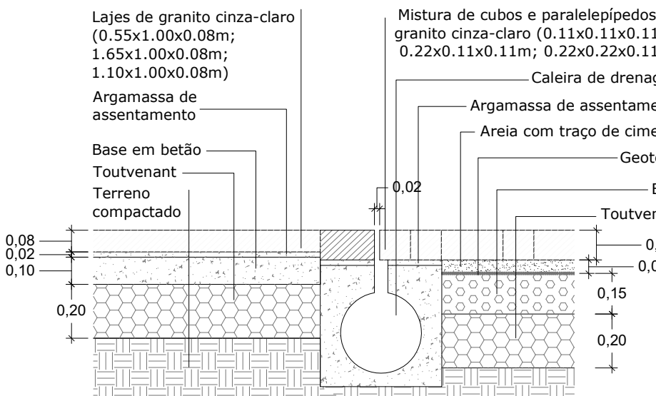
P12 - Alinhamento de paralelepípedos de granito cinza-escuro e caleira de drenagem (ver projecto de especialidade) entre pavimento automóvel e pedonal composto por mistura de cubos e paralelepípedos de granito cinza-claro e pavimento automóvel ligeiro e pedonal em lajes de granito cinza-claro de grandes dimensões Corte transversal
