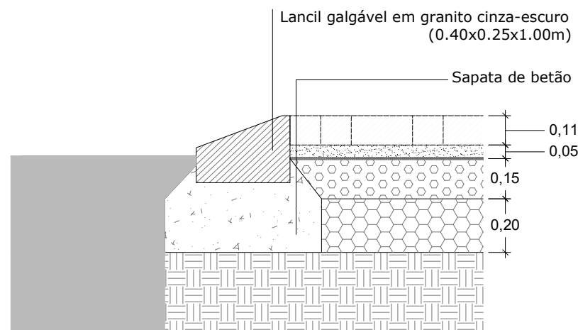
P2 - Remate em lancis galgáveis de granito cinza-escuro entre via existente exterior ao lote e pavimento automóvel e pedonal composto por mistura de cubos e paralelepípedos de granito cinza-claro Corte transversal
