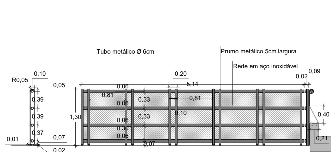
P45 - Portão 3 de correr em prumos e tubos metálicos, com revestimento em rede em aço inoxidável.
