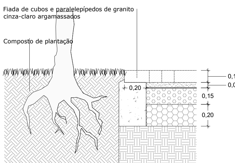
P5 - Remate em cubos e paralelepípedos de granito argamassados entre pavimento automóvel e pedonal composto por mistura de cubos e paralelepípedos de granito cinza-claro e caldeira Corte transversal
