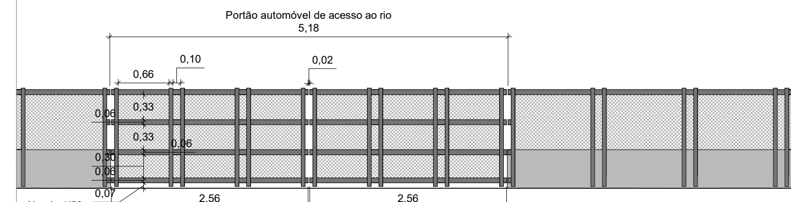
P47 - Portão 5 de abrir em prumos e tubos metálicos, com revestimento em rede em aço inoxidável.
