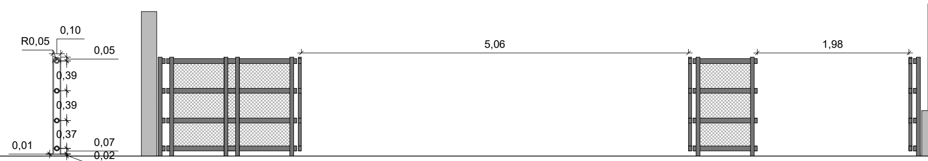
P43 - Portão 1 e porta de homem 2 de abrir em prumos e tubos metálicos, com revestimento em rede em aço inoxidável - portões abertos.
