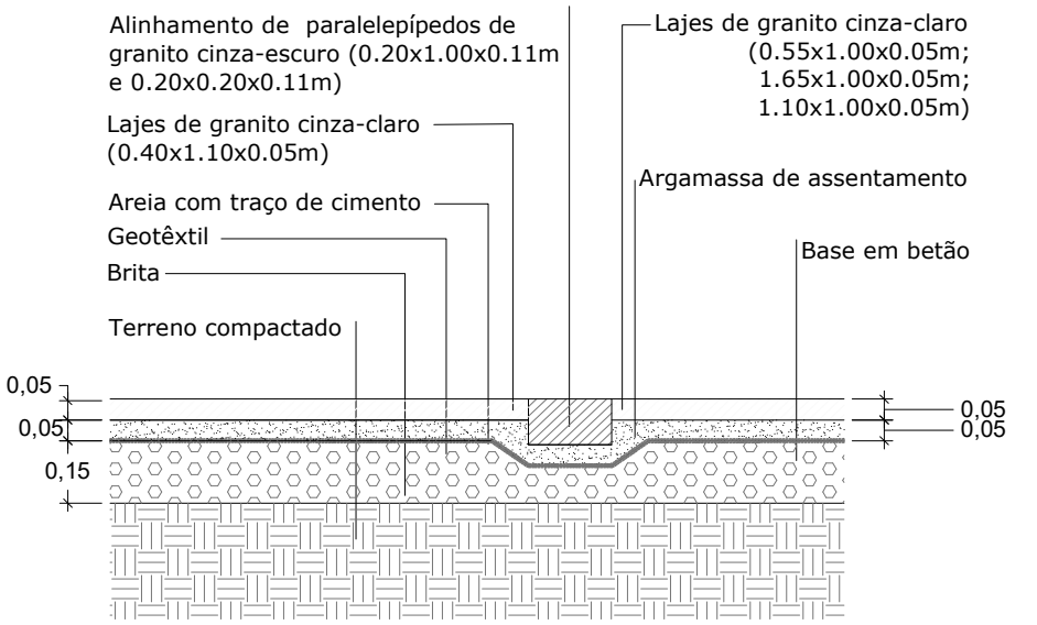
P19 - Alinhamento de paralelepípedos de granito cinza-escuro entre pavimentos pedonais em lajes de granito cinza-claro (0.40x1.10x0.08m e 0.55x1.00x0.08m; 1.65x1.00x0.08m; 1.10x1.00x0.08m) Corte transversal
