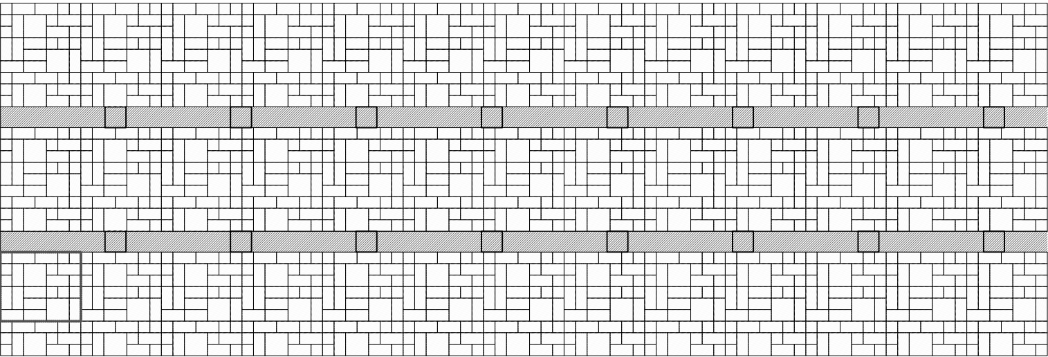
P 38 - Estereotomia do pavimento automóvel e pedonal composto por mistura de cubos e paralelepípedos de granito cinza-claro (0.11x0.11x0.11m; 0.22x0.11x0.11m; 0.22x0.22x0.11m), com alinhamentos de paralelepípedos de granito cinza-escuro (0.20x1.00x0.11m e 0.20x0.20x0.11m) Planta 1/50
