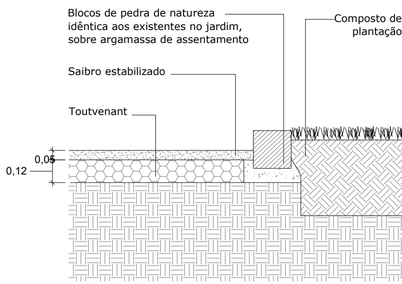
P24 - Remate em pedra, de natureza idêntica aos existentes no jardim, entre pavimento em saibro e zona verde Corte transversal
