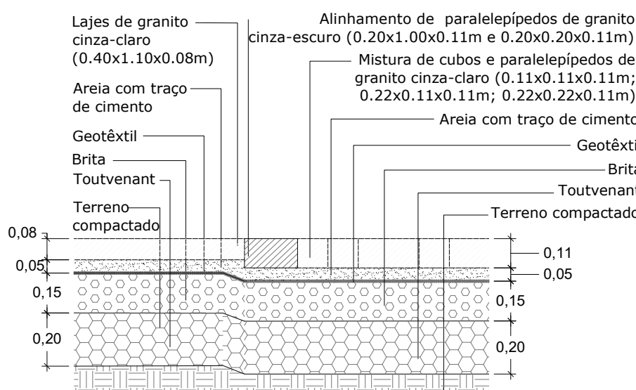
P11 - Alinhamento de paralelepípedos de granito cinza-escuro entre pavimento automóvel e pedonal composto por mistura de cubos e paralelepípedos de granito cinza-claro e pavimento automóvel ligeiro e pedonal em lajes de granito cinza-claro (0,40x1,00x0,08m) Corte transversal
