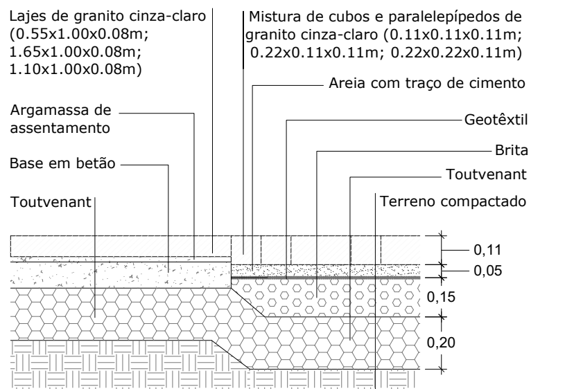
P8 - Remate entre pavimento automóvel e pedonal composto por mistura de cubos e paralelepípedos de granito cinza-claro e pavimento automóvel ligeiro e pedonal em lajes de granito cinza-claro Corte transversal
