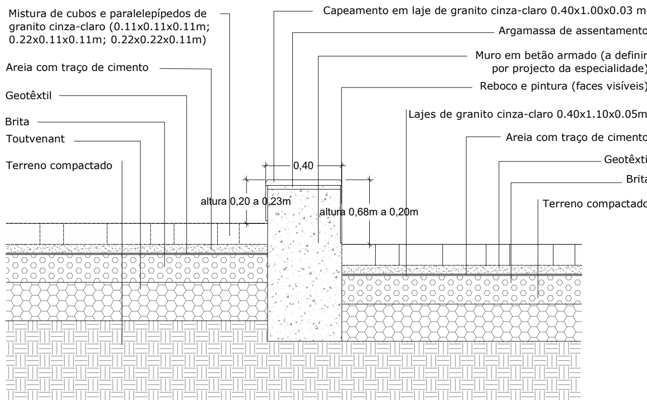
P35 - Muro de prolongamento do grande muro existente. Corte transversal
