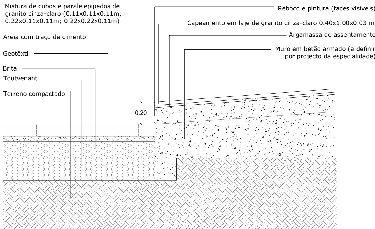
P35 - Muro de prolongamento do grande muro existente. Corte longitudinal
