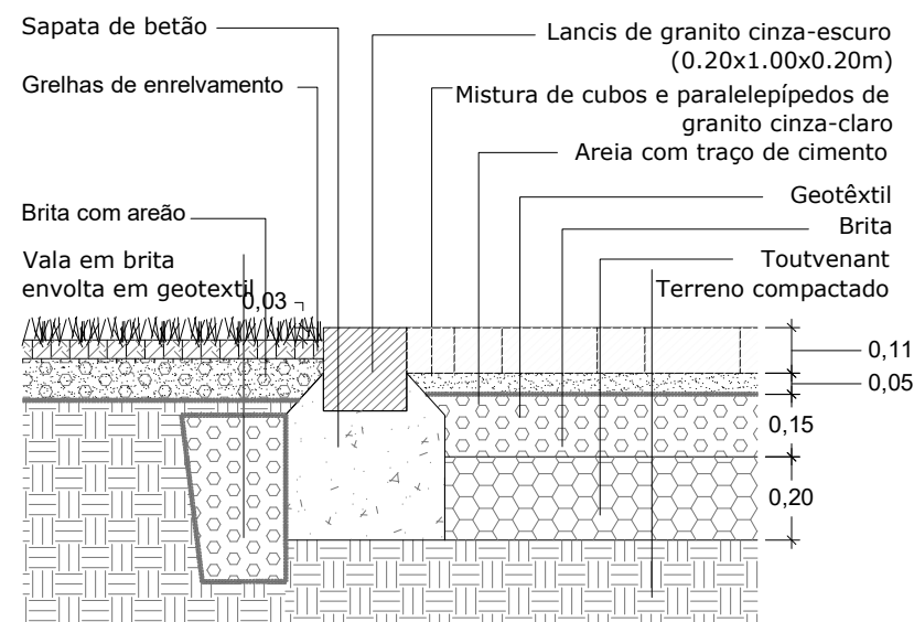
P4 - Remate contínuo em lancis de granito cinza-escuro entre estacionamento eventual em grelhas de enlhecimento e pavimento automóvel e pedonal composto por mistura de cubos e paralelepípedos de granito cinza-claro Corte transversal
