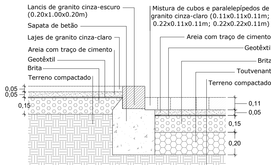
P10 - Remate em lancis de granito cinza-escuro entre pavimento automóvel e pedonal composto por mistura de cubos e paralelepípedos de granito cinza-claro e pavimento pedonal em lajes de granito cinza-claro Corte transversal
