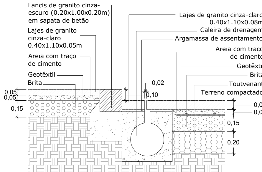
P14 - Remate em lancis de granito cinza-escuro e caleira de drenagem (ver projecto da especialidade) entre pavimento automóvel ligeiro e pedonal em lajes de granito cinza-claro (0.40x1.10x0.08m) e pavimento exclusivamente pedonal em lajes de granito cinza-claro (0.40x1.10x0.05m) Corte transversal
