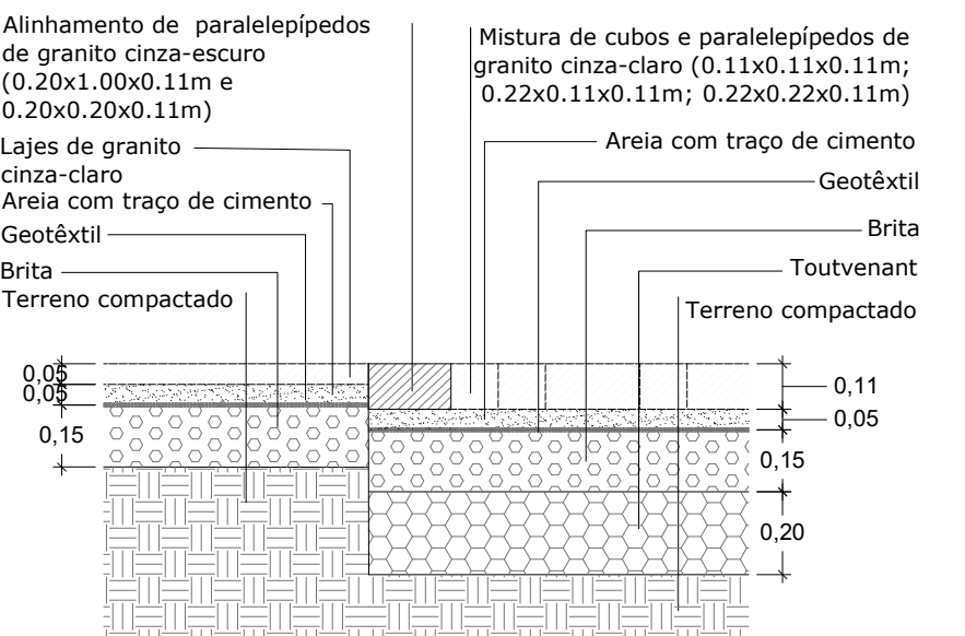
P9 - Alinhamento de paralelepípedos de granito cinza-escuro entre pavimento automóvel e pedonal composto por mistura de cubos e paralelepípedos de granito cinza-claro e pavimento pedonal em lajes de granito cinza-claro Corte transversal
