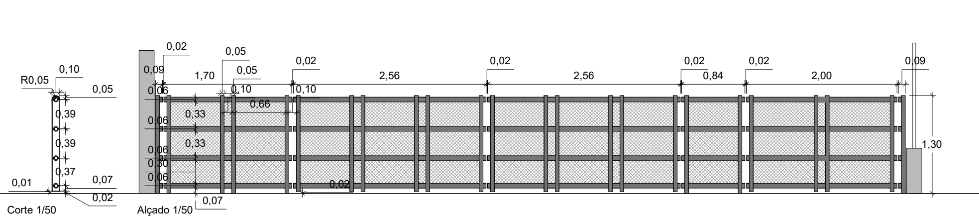
P43 - Portão 1 e porta de homem 2 de abrir em prumos e tubos metálicos, com revestimento em rede em aço inoxidável - portões fechados.
