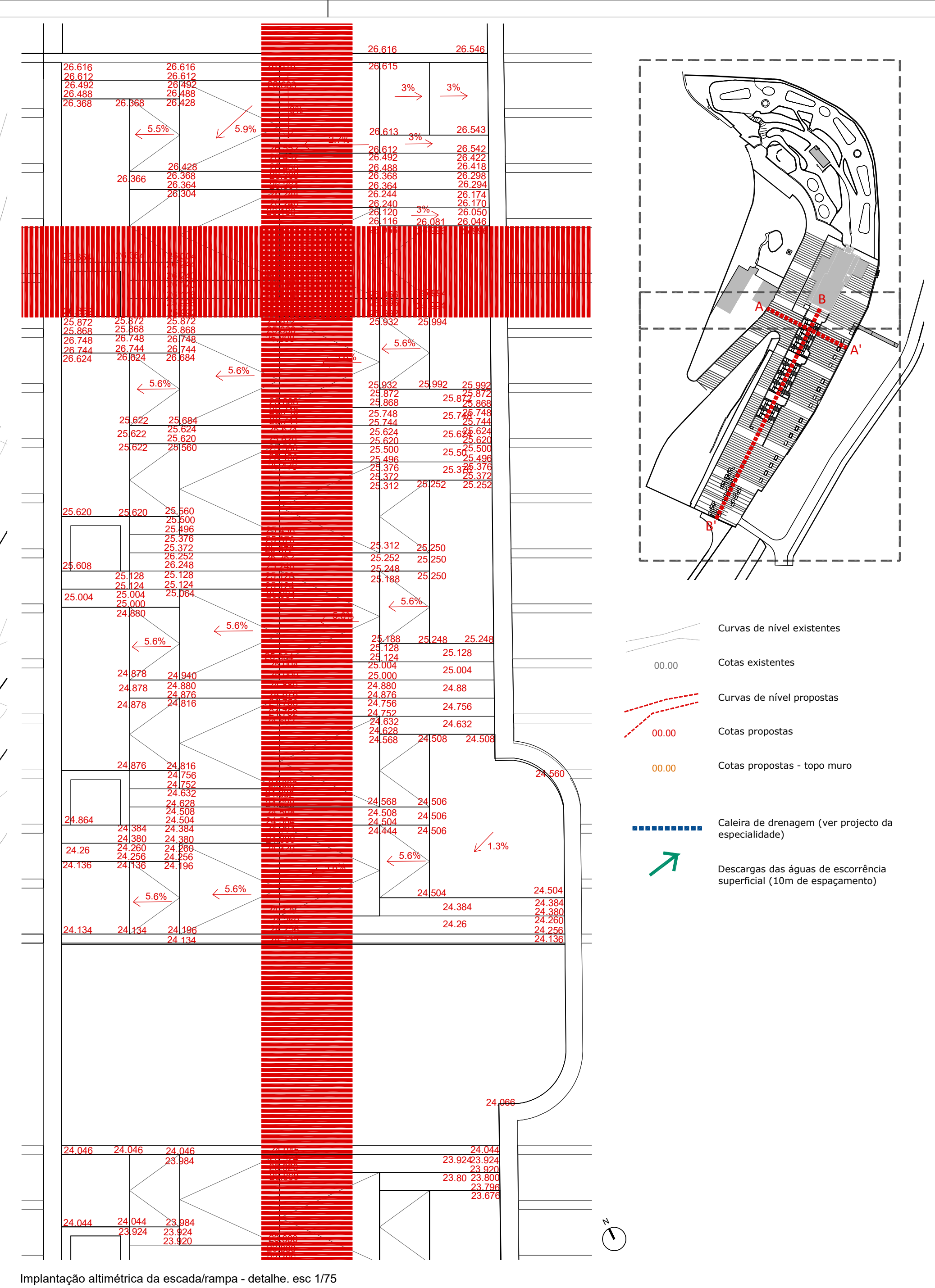
Implantação altimétrica da escada/rampa - detalhe, esc. 1/75
