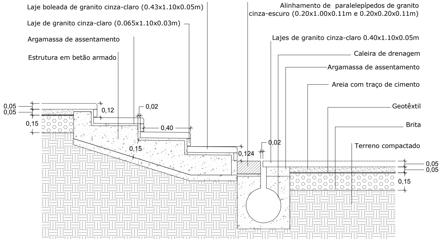
P27 - Alinhamento de paralelepípedos de granito cinza-escuro e caleira de drenagem entre degraus revestidos a lajes de granito cinza-claro e patamares em lajes de granito cinza-claro de 0.40x1.10x0.05m Corte transversal
