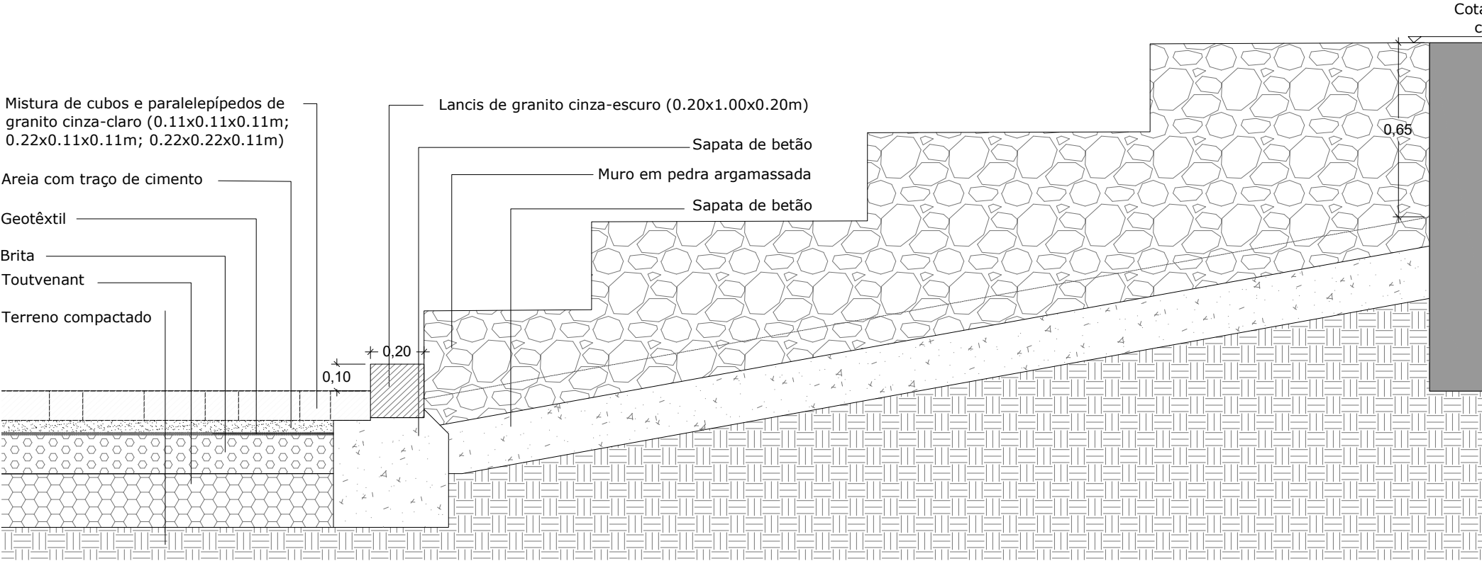
P37 - Muro em pedra no talude. Corte longitudinal 1/20
