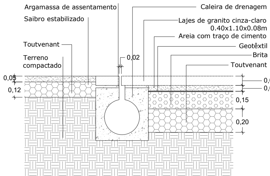
P21 - Caleira de drenagem entre pavimento automóvel ligeiro e pedonal em lajes de granito cinza-claro de 0.40x1.10m e pavimento em saibro Corte transversal
