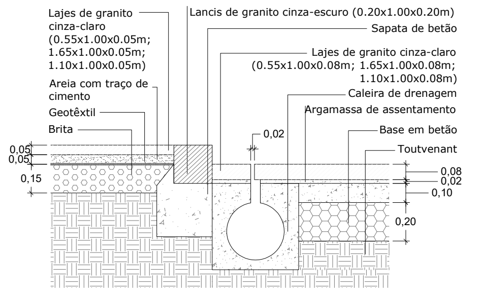
P15 - Remate em lancis de granito cinza-escuro e caleira de drenagem (ver projecto da especialidade) entre pavimento automóvel ligeiro e pedonal em lajes de granito cinza-claro de grandes dimensões e pavimento exclusivamente pedonal em lajes de granito cinza-claro de grandes dimensões Corte transversal
