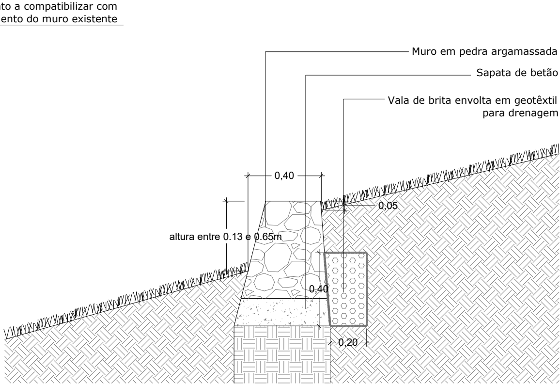
P37 - Muro em pedra no talude. Corte transversal 1/20
