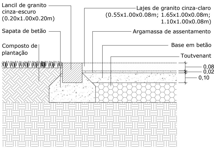
P17 - Remate entre pavimento automóvel ligeiro e pedonal em lajes de granito cinza-claro de grandes dimensões e zona verde Corte transversal
