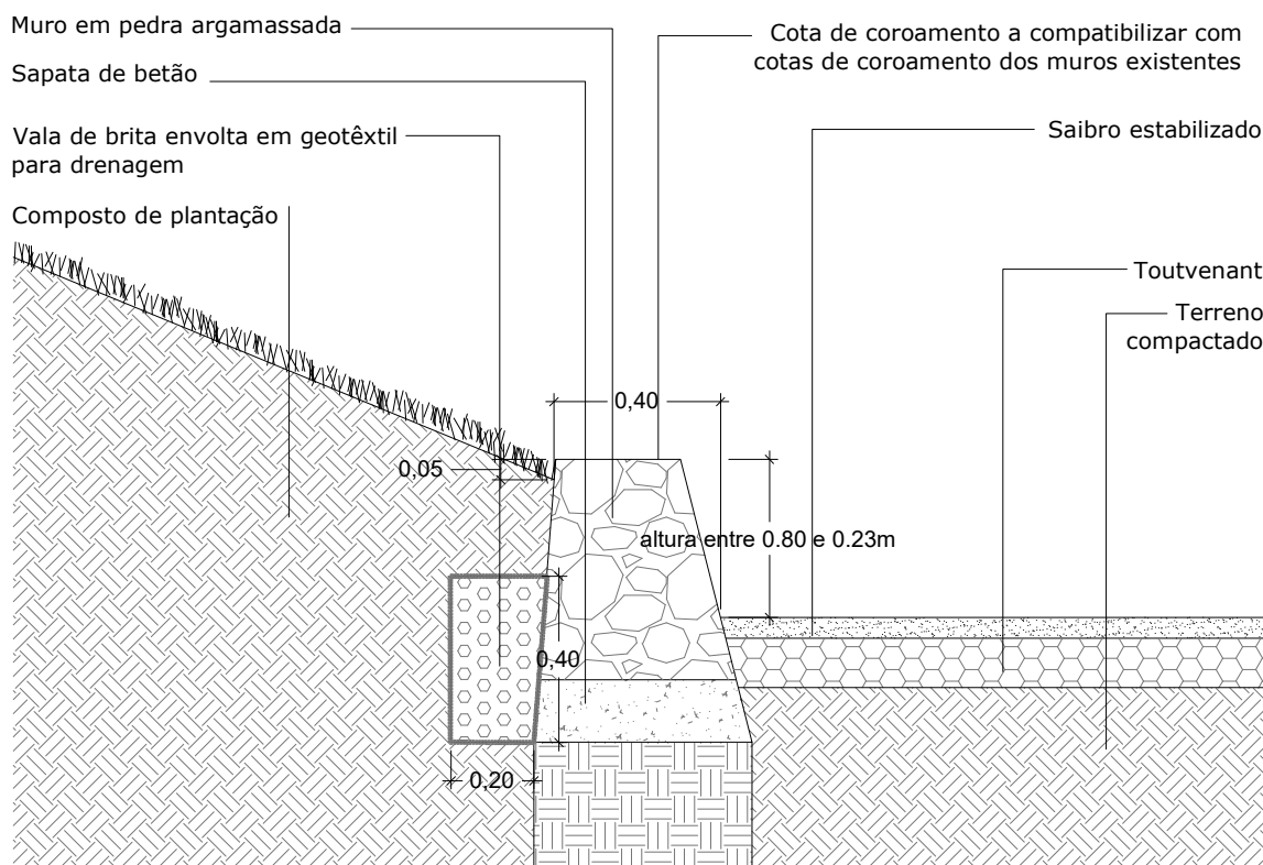
P36 - Muro em pedra no Jardim da Rocha Corte transversal
