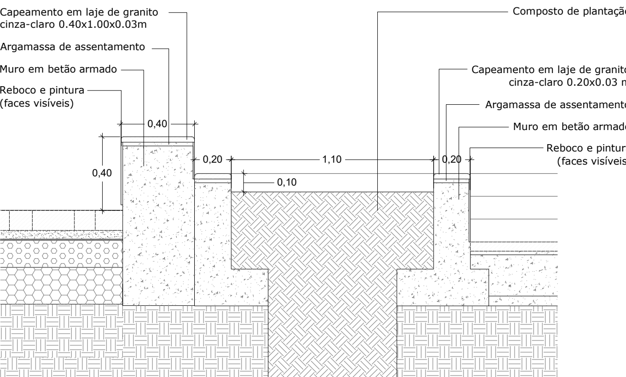
P29 - Caldeira para árvore, encaixada na escada, capeada a lajes de granito cinza-claro e muro de remate entre escada/rampa de acesso à Igreja e a faixa automóvel . Corte
